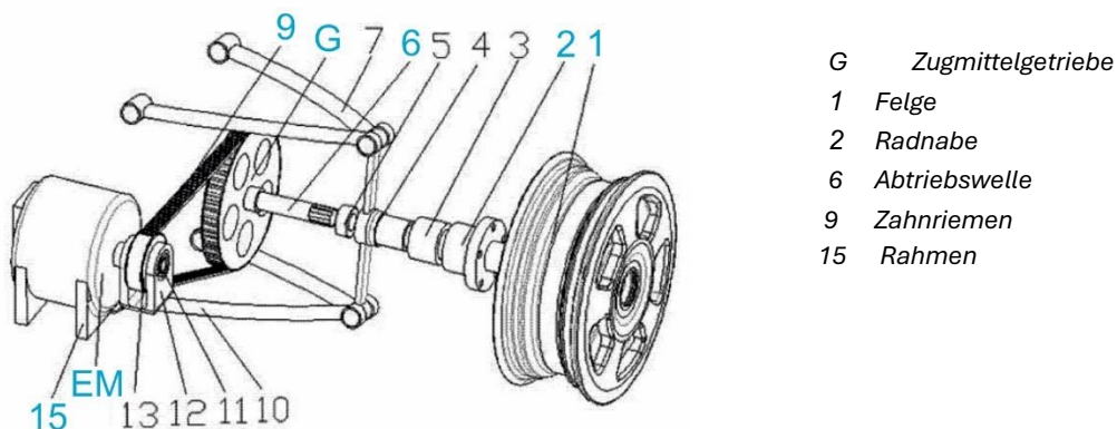
Abb. 4.35: Paralleler Einzelradantrieb aus CN 203832232 U (Fig. 1) angemeldet am 14.04.2014
