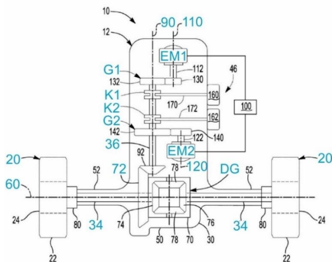
Abb. 4.6: Winkelantrieb aus EP 4292855 A2 (Fig. 1) angemeldet am 21.01.2021
