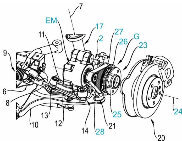
Abb. 4.62: Paralleler Radnabenantrieb aus DE 102022202016 B3 (Fig. 2) angemeldet am 28.02.2022
