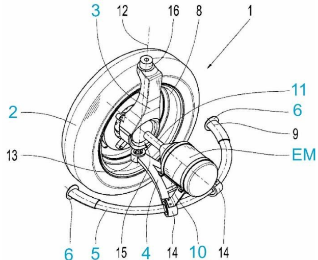
Abb. 4.46: Direktantrieb aus DE 102015226589 A1 (Fig. 1) angemeldet am 22.12.2015
