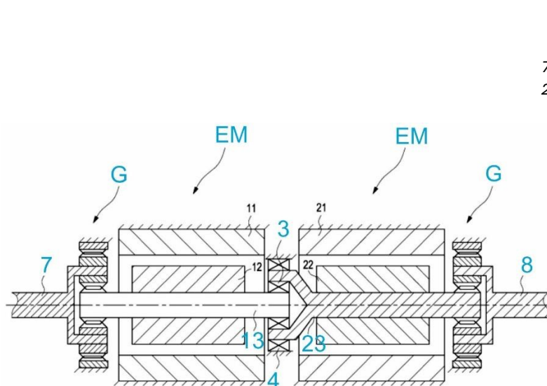
Abb. 4.36: Koaxialer Einzelradantrieb aus DE 102016222844 A1 (Fig. 1) angemeldet am 21.11.2016
