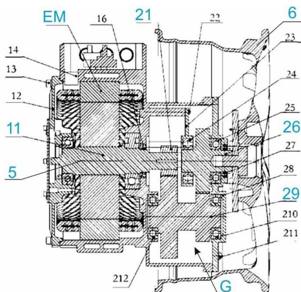
Abb. 4.58: Koaxialer Radnabenantrieb aus CN 110203058 A (Fig. 2) angemeldet am 31.05.2019
