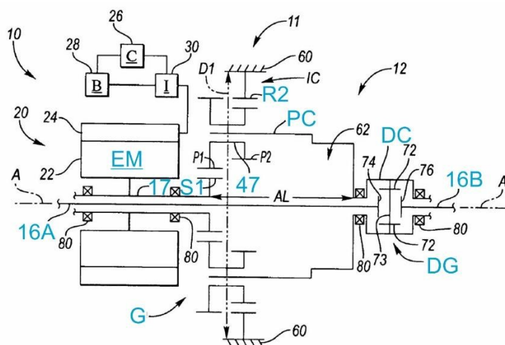
Abb. 4.20: Koaxialantrieb aus DE 102015106503 A1 (Fig. 1) angemeldet am 28.04.2015
