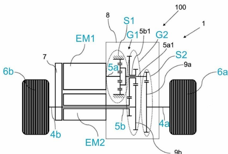
Abb. 4.39: Koaxialer Einzelradantrieb aus DE 102021211660 A1 (Fig. 3) angemeldet am 15.10.2021
