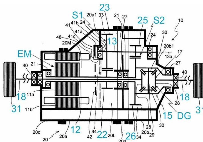
Abb. 4.21: Koaxialantrieb aus DE 102015016636 A1 (Fig. 1) angemeldet am 21.12.2021
