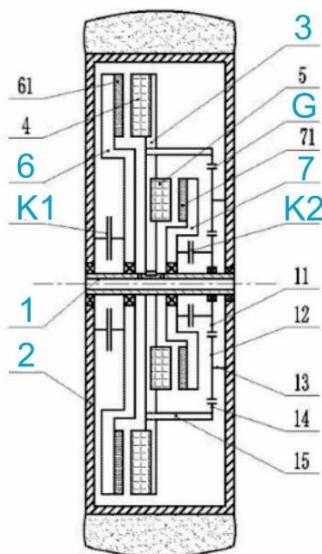
Abb. 4.60: Koaxialer Radnabenantrieb aus GB 2599592 A (Fig. 1) angemeldet am 16.03.2021
