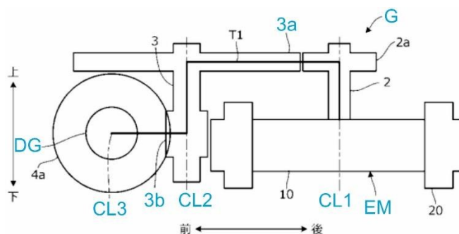
Abb. 4.3: Winkeltrieb aus JP 2019115135 A (Fig. 1) angemeldet am 22.12.2017
